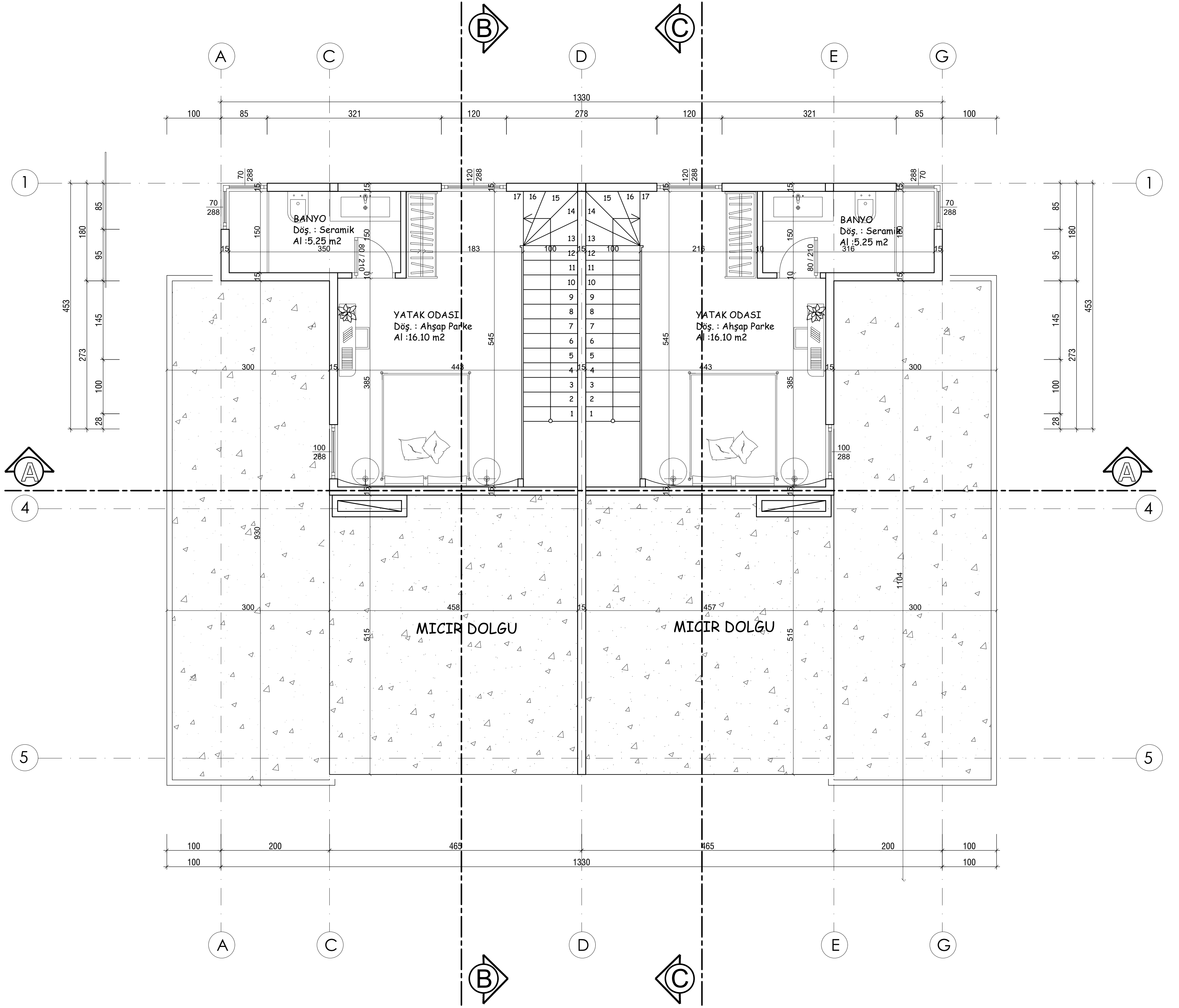
B BLOK TİP LOFT KAT PLANI
