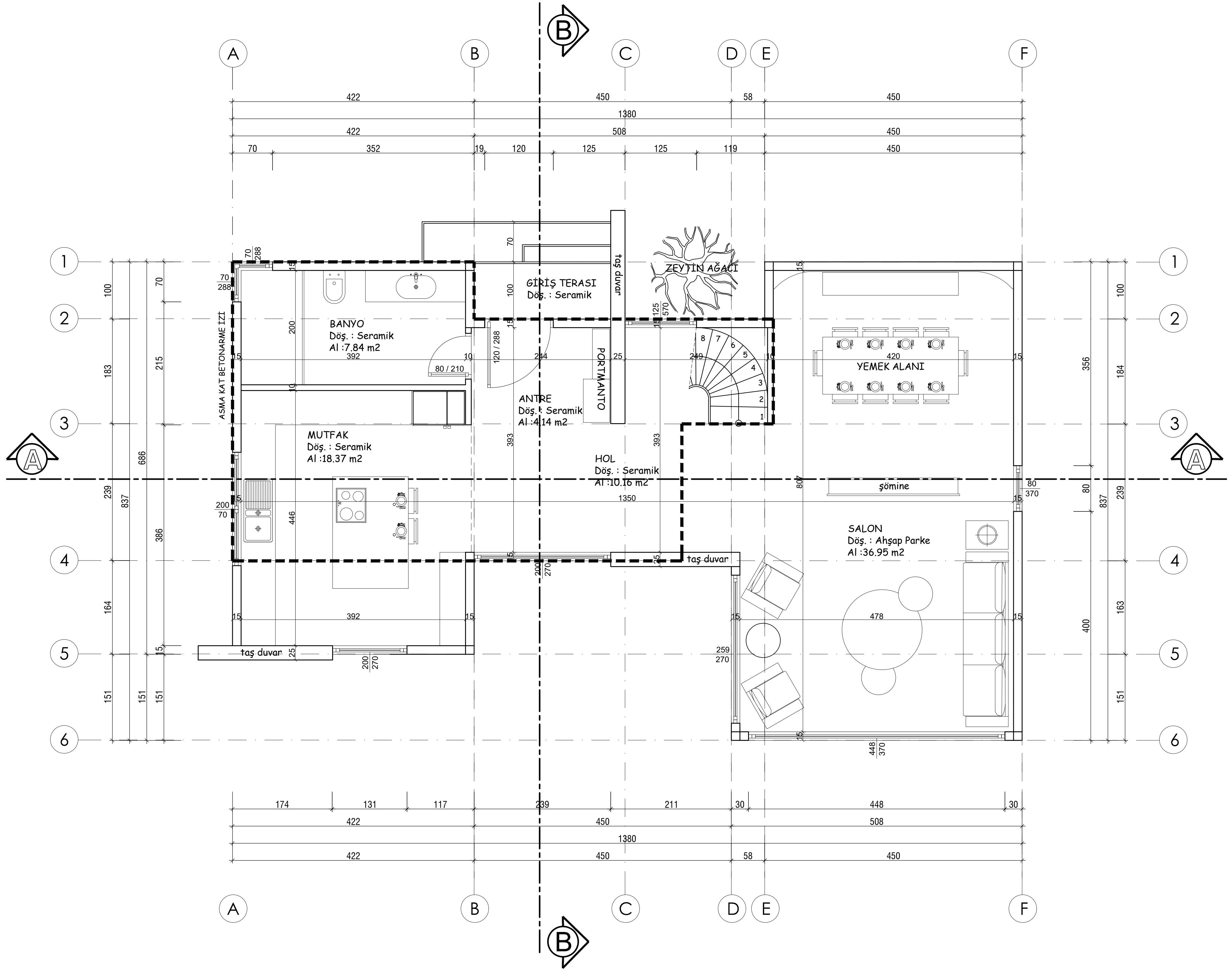
A BLOK ZEMİN KAT PLANI
